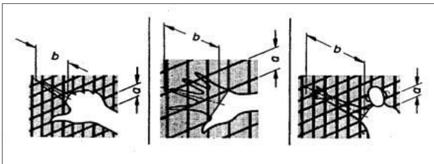
a=Öffnungsweite; b=Sicherheitsabstand
