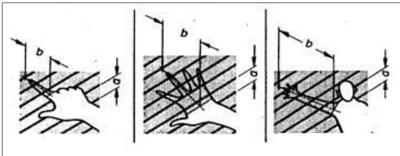
a=Öffnungsweite; b=Sicherheitsabstand
