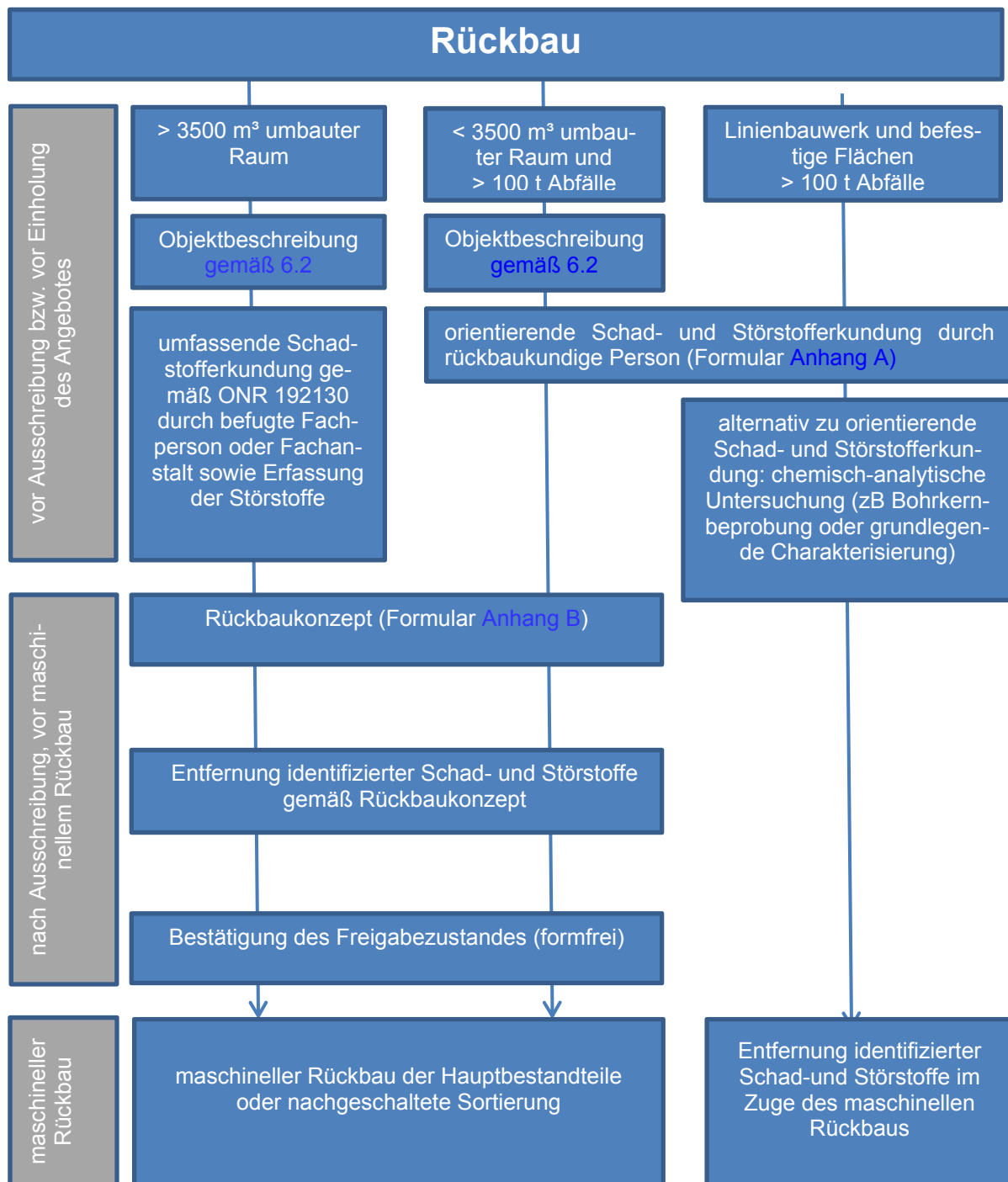
Bild C.1 — Rückbau
