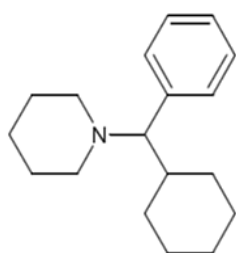
1-[Cyclohexyl(Phenyl)methyl]-Piperidin
