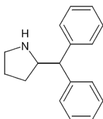
1-[Cyclohexyl(Phenyl)methyl]-Piperidin
