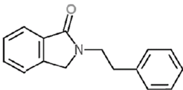
2-(Phenyl ethyl)-3H-Isoindol-1-on
