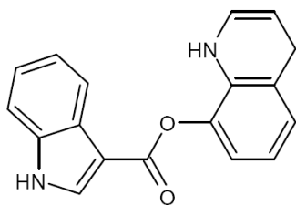
Indol-3-Carbonsäure-8-Quinolinylderivat
