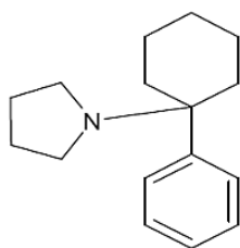
1-(1-Phenylcyclohexyl)-Pyrrolidin
