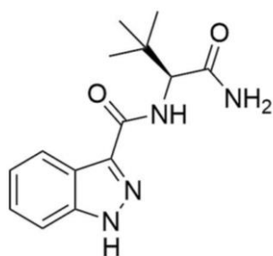
N-(1-Amino-3,3-Dimethyl-1-Oxo-2-Butanyl)-1H- Indazol-3-Carboxamid
