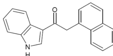
1-(1H-Indol-3-yl)-2-(Naphthalen-1-yl)-Ethanon
