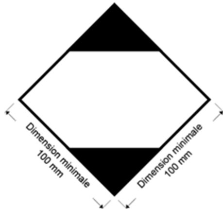
Marquage des colis contenant des quantités limitées
