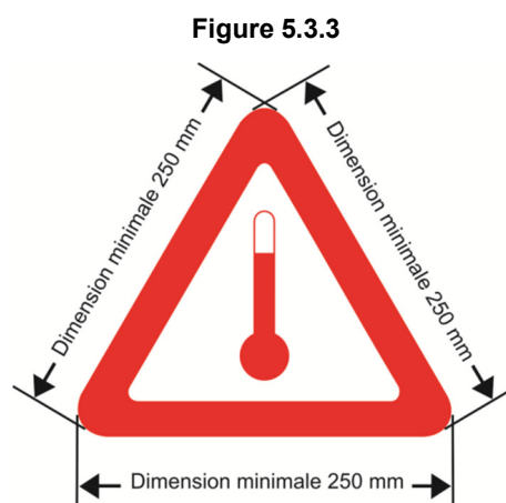
Marque pour les matières transportées à chaud
