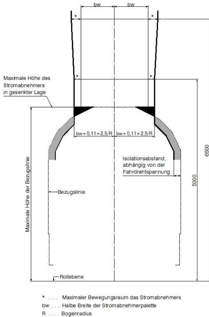
Bild 4: Bezugslinie für Stromabnehmer (Maße in mm)
