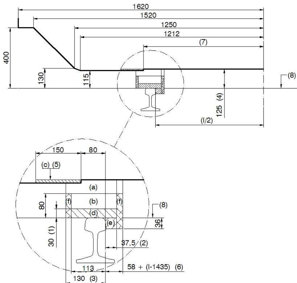
Bild 2: Unterer Teil der Bezugslinie für Schienenfahrzeuge, die Gleisbremsen in Bremsstellung oder sonstige aktivierte Verschub- oder Abbremsvorrichtungen befahren dürfen. (Maße in mm)
